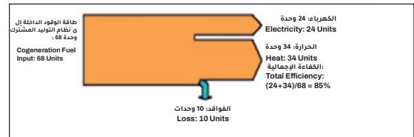
إمداد الطاقة بالتوليد المشترك / ENERGY SUPPLY WITH COGENERATION
