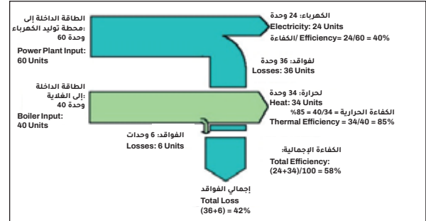
إمداد الطاقة بالطريقة التقليدية / CONVENTIONAL ENERGY SUPPLY
