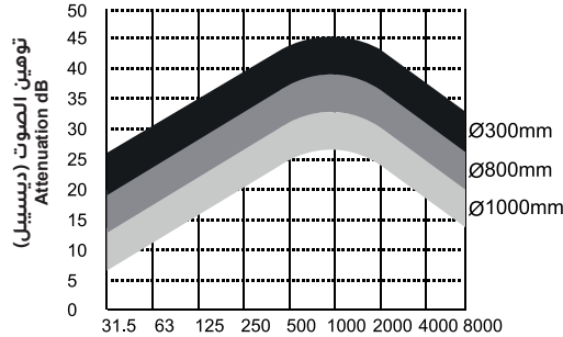
منحنى توهين الصوت (ديسيبل) ATTENUATION GRAPH (dB)
