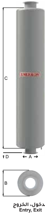
الرسم المرجعي للأبعاد DIMENSION REFERENCE DIAGRAM
